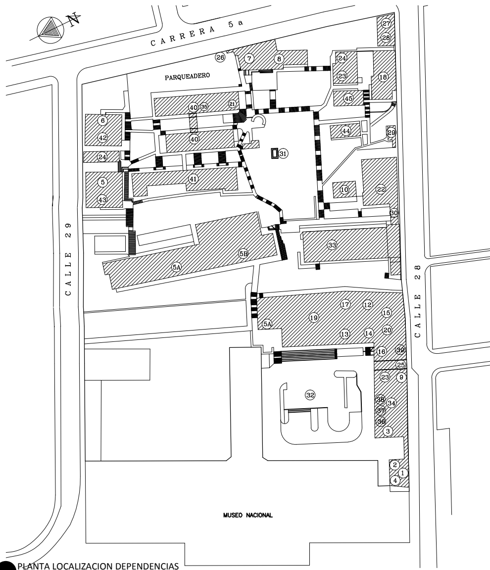
PLANTA LOCALIZACION DEPENDENCIAS ESC 1:1500
